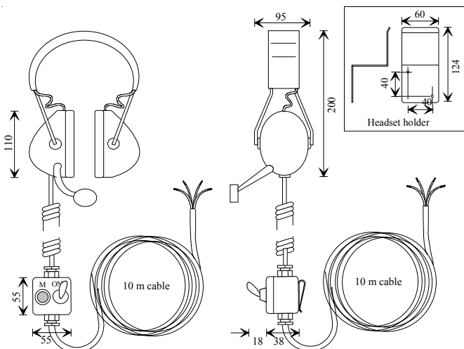
Headset holder (wall bracket)
